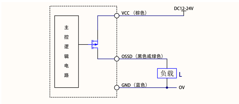
图 6-9 MC-C1 安全光幕 PNP 输出波形
