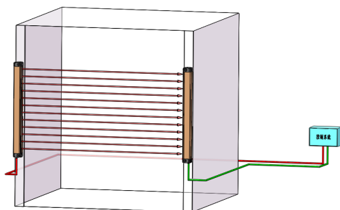
图 3-2 线同步方式
