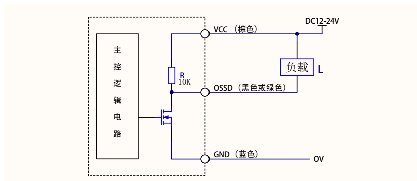
图6-2 MC安全光幕NPN输出结构图
