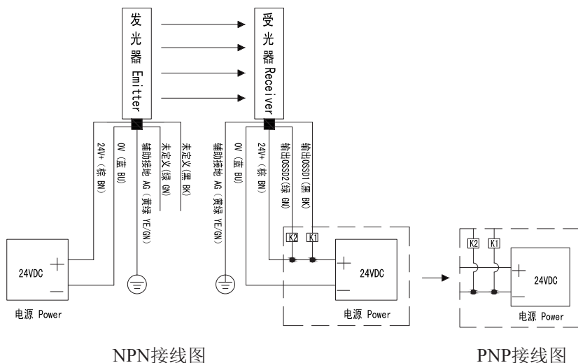
图 6-1 MC 系列安全光幕接线图
