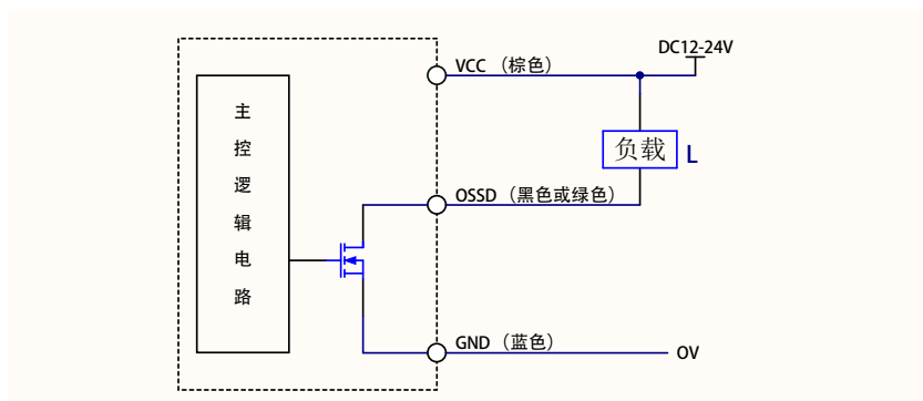
图6-5 MC-C安全光幕NPN输出结构图
