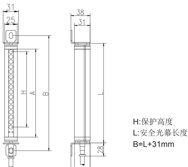
图4-3 MC系列安全光幕外形尺寸图
