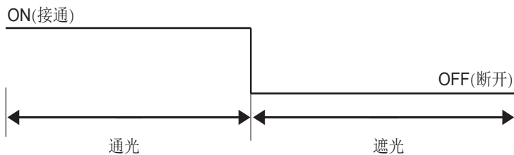
图 6-11 MC-C1 安全光幕输出（黑色线）波形
