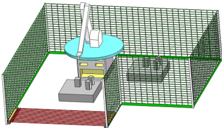
图3-5 使用MC系列安全光幕的危险区域保护
