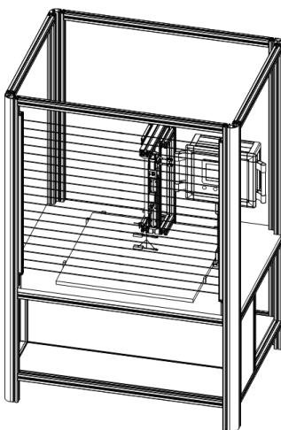
图3-4 使用MC系列安全光幕的危险点保护
