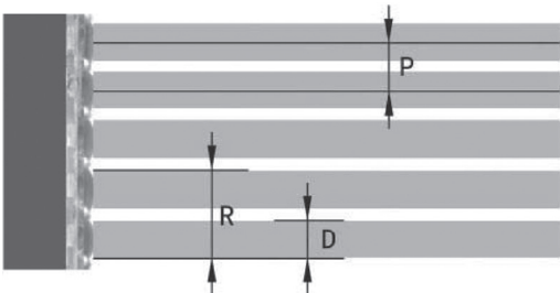
图3-1 检测精度与光轴间距的关系 P为光轴间距，R为检测精度，D为透镜尺寸； R=P+D ;
