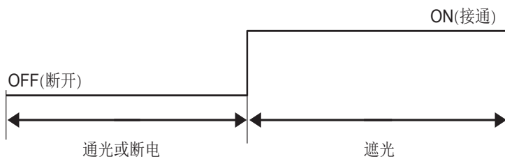
图 6-14 MC-C2 安全光幕输出波形
