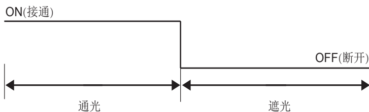
图 6-7 MC-C 安全光幕输出波形
