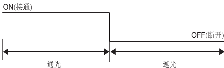
图 6-4 MC 安全光幕输出波形
