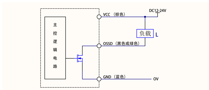
图6-8 MC-C1安全光幕NPN输出结构图
