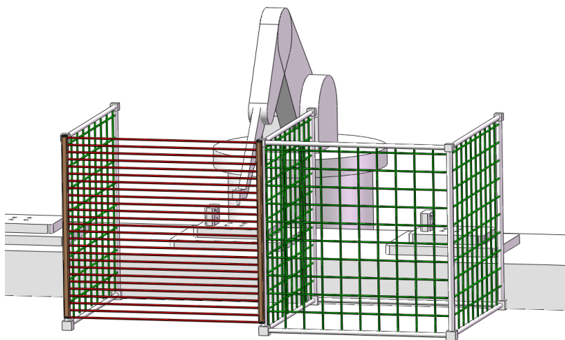
图3-6 使用MC系列安全光幕的进入保护
