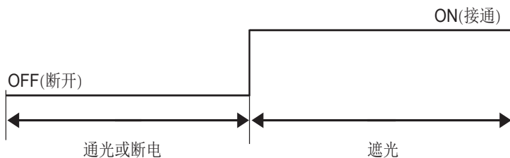
图 6-10 MC-C1 安全光幕输出（绿色线）波形
