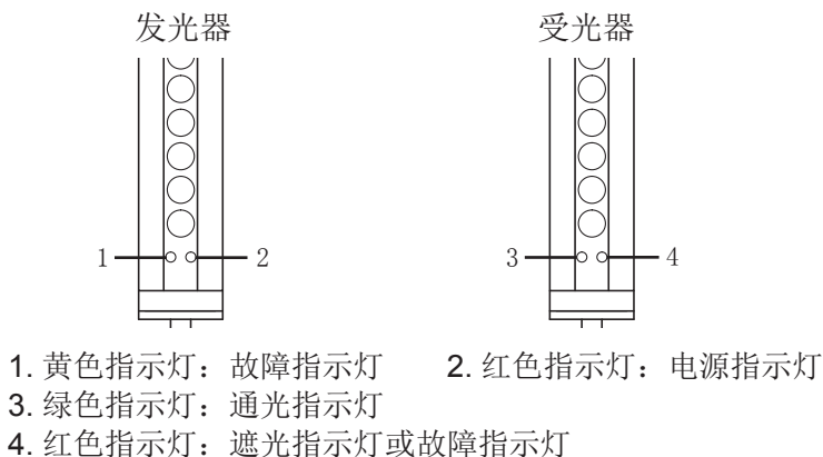
图4-2 MC系列安全光幕指示灯图
