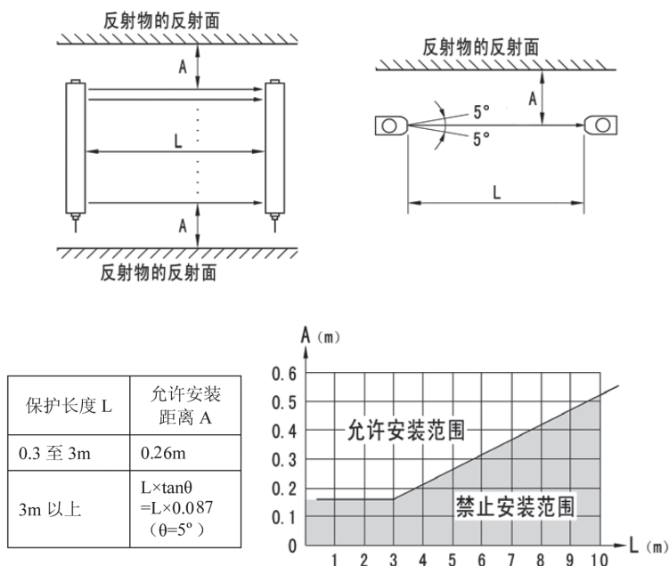
图5-7 防止周围反射物对光幕产生影响的安装位置示意图
