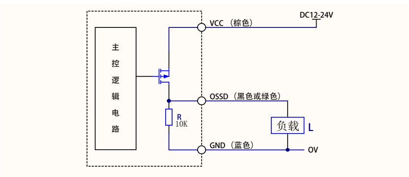
图 6-3 MC 安全光幕 PNP 输出结构图
